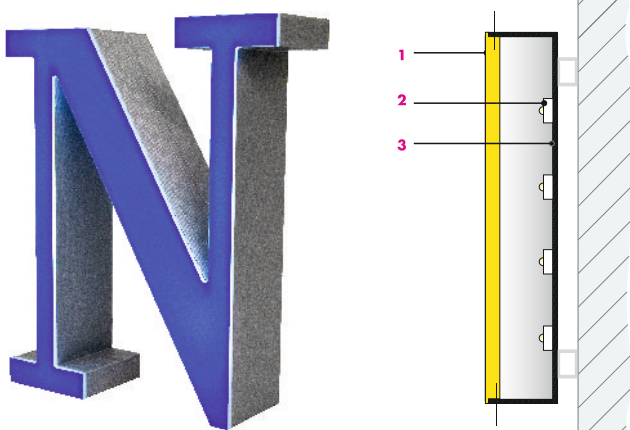
1 Acrylglasfront 2 LED-Modul 3 Untergehäuse 3Dprint
