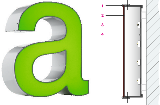
1 PVC-Umleimer 2 Acrylglasfront 3 LED-Modul 4 Untergehäuse
