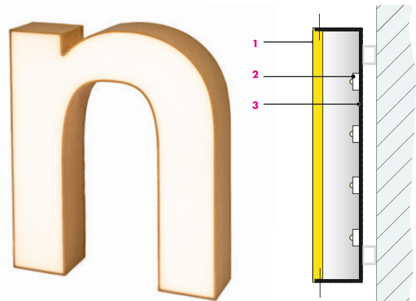
1 Acrylglasfront 2 LED-Modul 3 Untergehäuse 3Dprint
