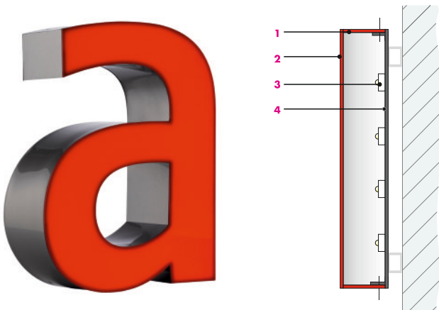
1 Acrylglaszarge, leuchtend 2 Acrylglasfront, deckend 3 LED-Modul 4 Alu-Boden
