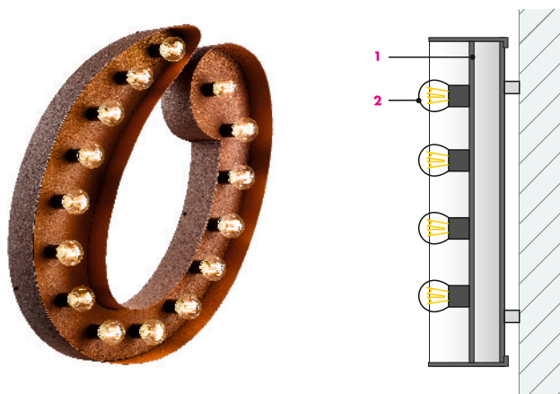
1 Alu-Gehäuse 2 LED-Glühlampe
