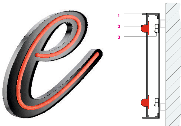
1 Alu-Gehäuse 2 Acrylglaskontur 3 LED-Modul
