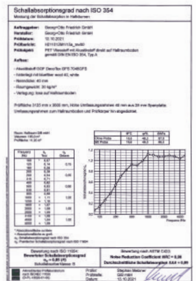
40mm Akustik-Vlies
