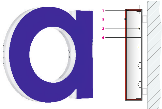
1 Acrylglaszarge, leuchtend 2 Acrylglasfront, leuchtend 3 LED-Modul 4 Alu-Boden
