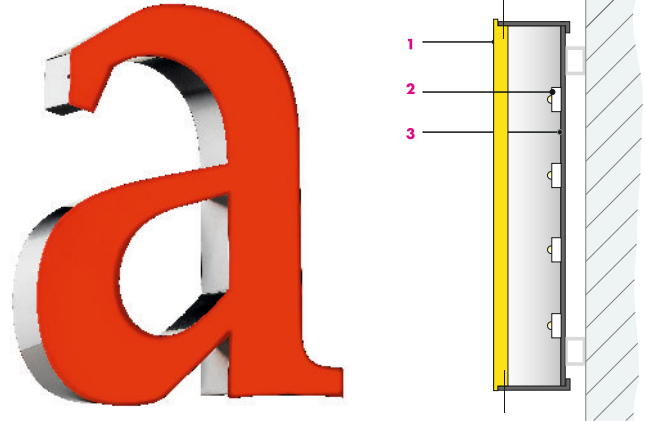
1 Acrylglasfront 2 LED-Modul 3 Untergehäuse
