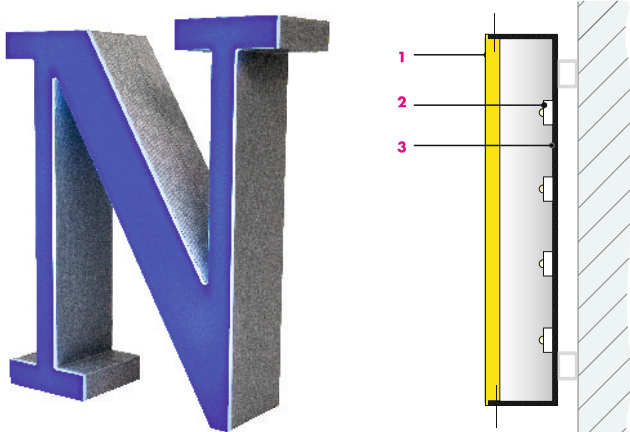
1 Acrylglasfront 2 LED-Modul 3 Untergehäuse 3Dprint
