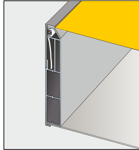
Schnittzeichnung Profil
